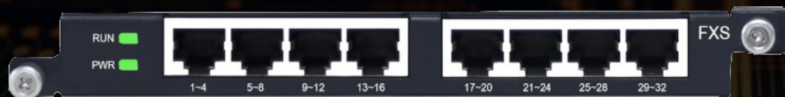
W&T-FXS32 (внутренних 32 аналоговых порта)
